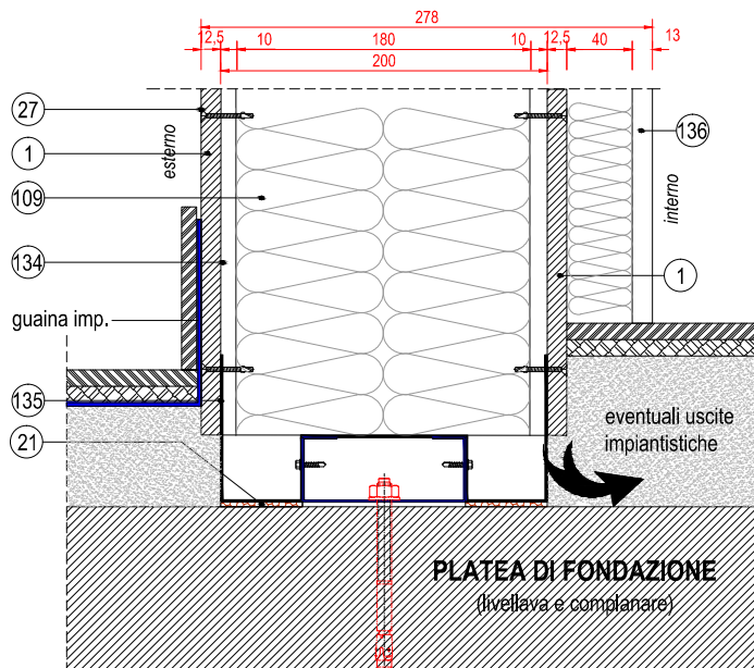
Sezione verticale su solaio
