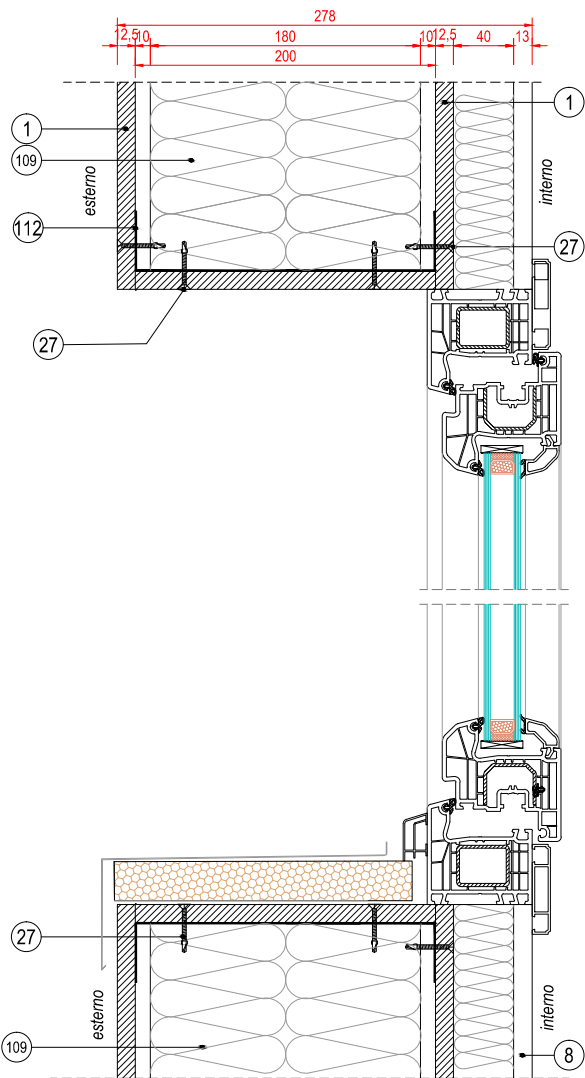
Sezione verticale su infisso
